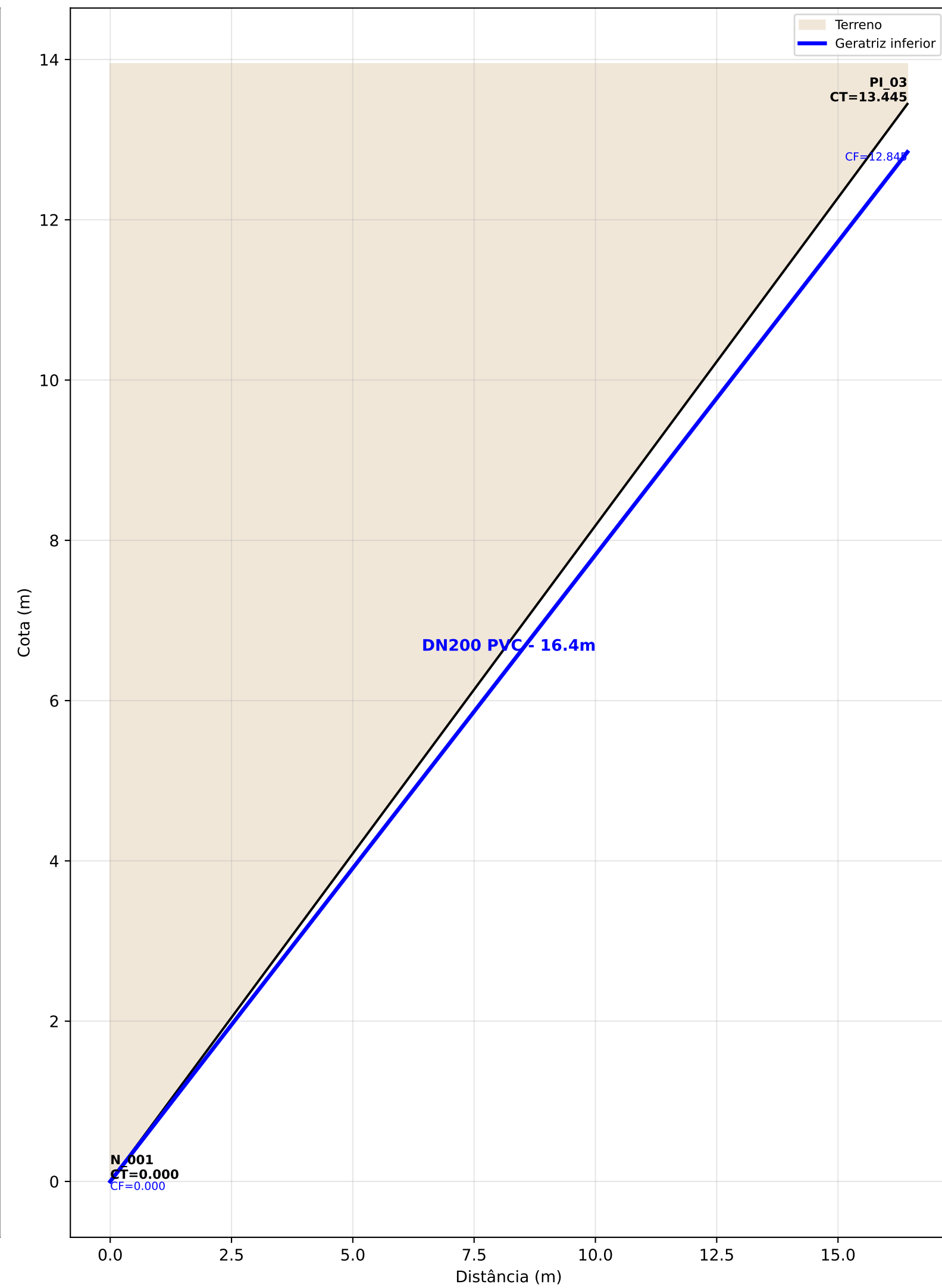
PERFIL LONGITUDINAL - NS 1
